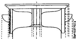
Նկ. 55. Բալյուստր
