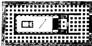
Նկ. 111. Դիպտերոն
