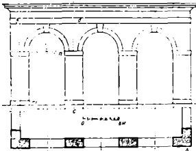
Նկ. 42. Արկադա
