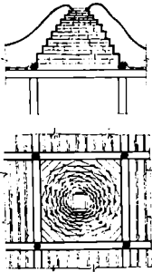
Նկ. 122. Երդիկավոր ծածկ
