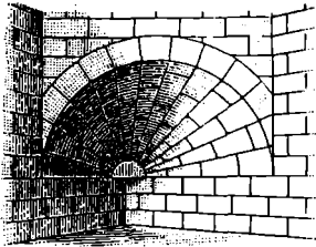
Նկ. 371. Տրոմպ
