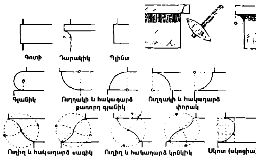
Նկ. 363. Տրամատ
