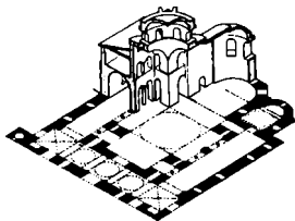
Նկ. 171. Խաչաձև զմբեթավոր եկեղեցի
