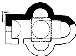
Նկ. 120. Եռախորան
