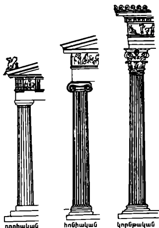
Նկ. 326. Սյունակարգ
