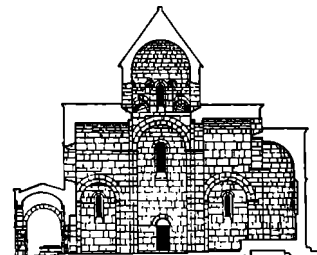
Նկ. 205. Կտրվածք ընդերկայնական
