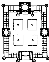
Նկ. 240. Մեդրեսե
