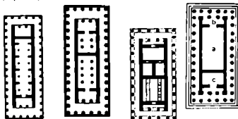
Նկ. 283. Պերիպտերոս
