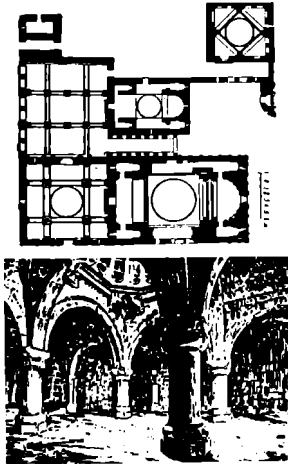
Նկ. 83. Գավիթ
