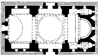
Նկ. 93. Գմբեթավոր դահլիճ
